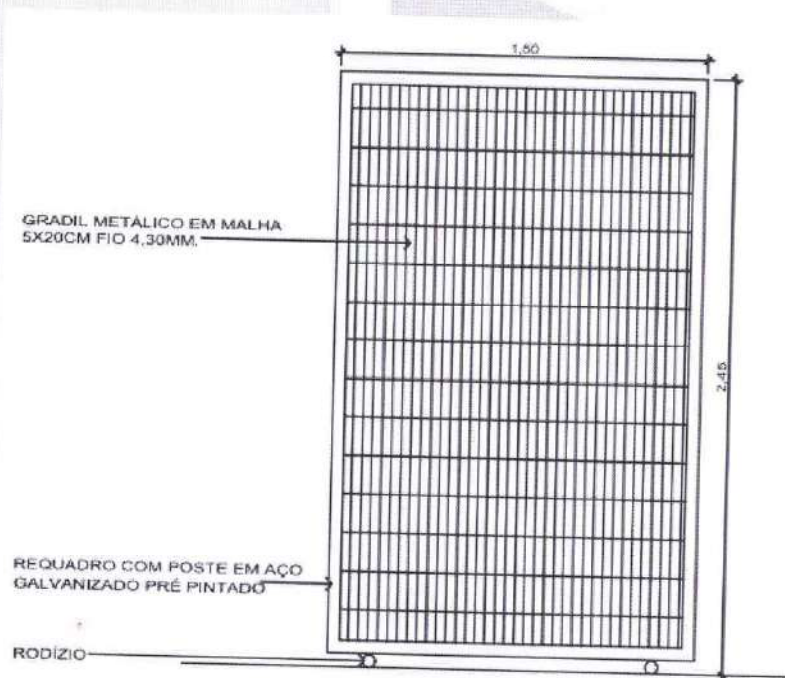
2 DETALHE PORTÃO 09 ESCALA 1:25
